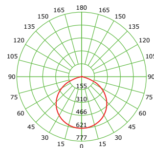
CURVA FOTOMETRICA
